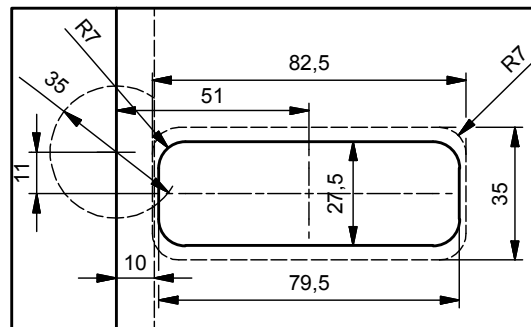
Milling groove / Fräsbild
